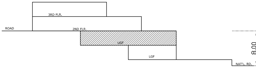
ELEVATION
