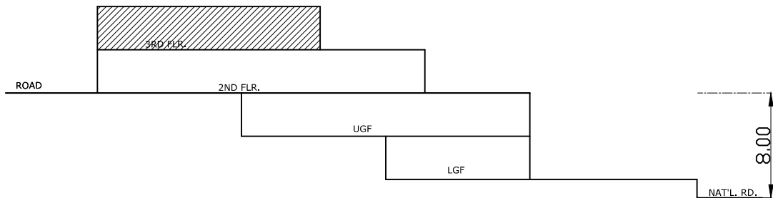
ELEVATION
